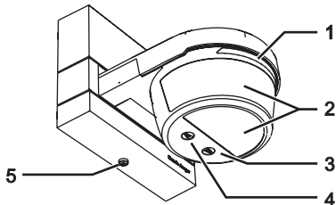
Abb. 17: Bedienelemente
