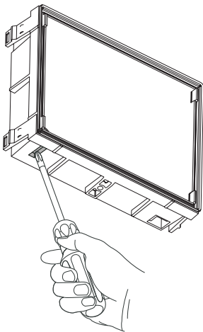
Abb. 8: Wasserablauf öffnen
